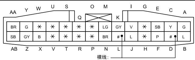
0922-202 巡航控制开关/ 巡航控制开关照明LH/ 巡航控制开关照明RH/ 巡航控制开关照明/ 转向开关照明/ 转向开关照明(综合信息显示屏)/ 转向开关/ 时钟弹簧/ 转向开关(综合信息显示屏)
